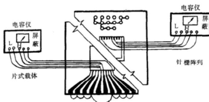
图1 引线间电容测试示意图
