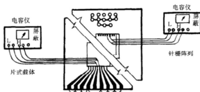
图2 引线负载电容测试示意图 2]
